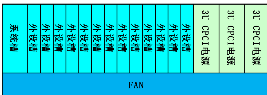
前视图
