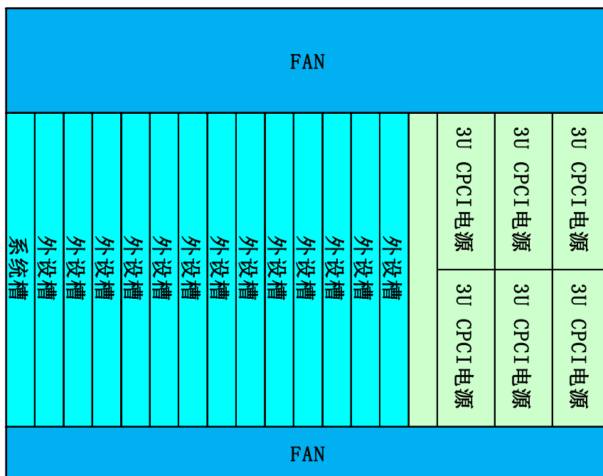
前视图
