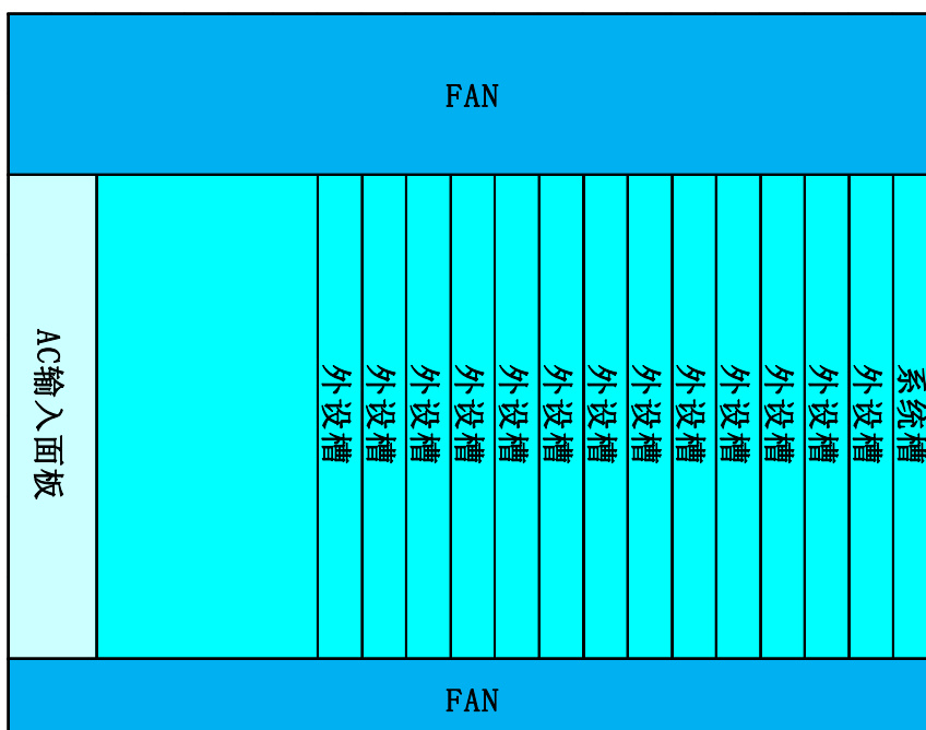
后视图
