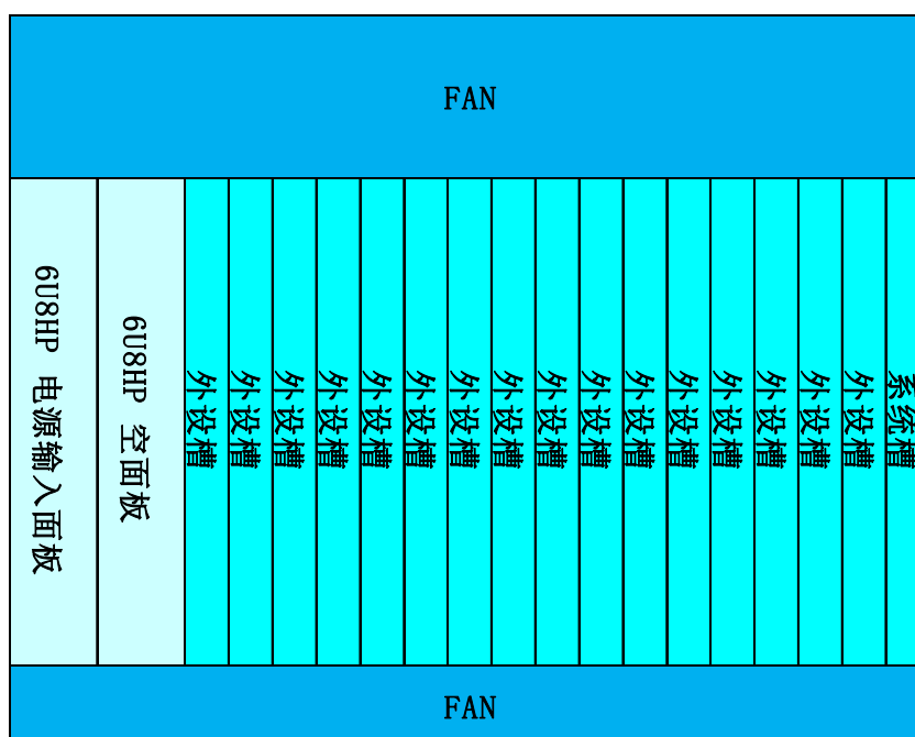
后视图
