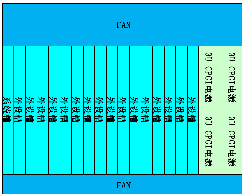
前视图
